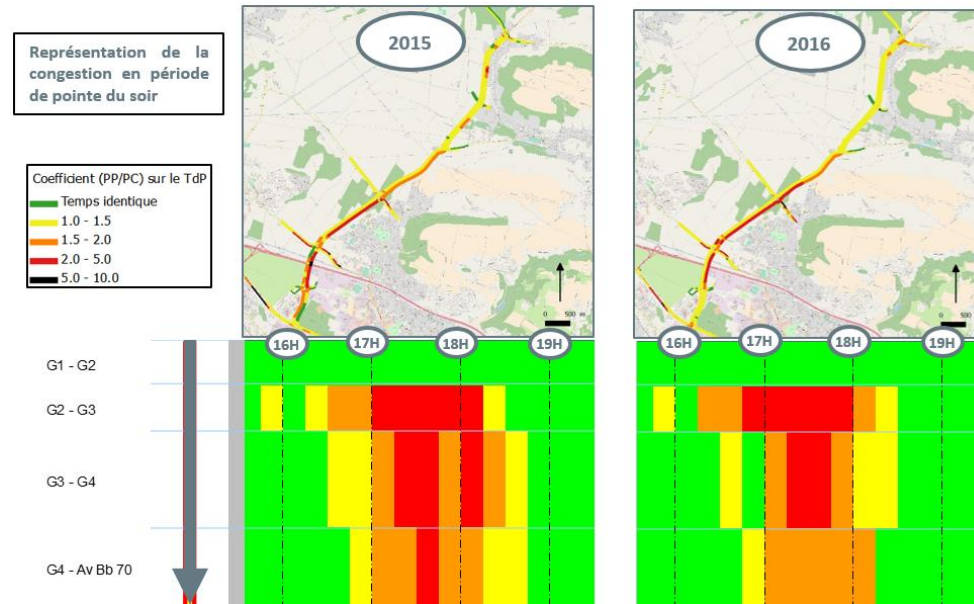
Exemple de graphique espace-temps montrant l'évolution d'une congestion entre 2015 et 2016
